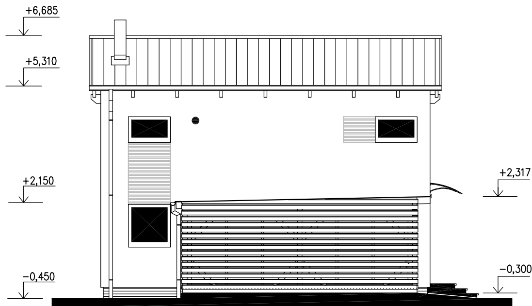
POHLED ULIČNÍ
