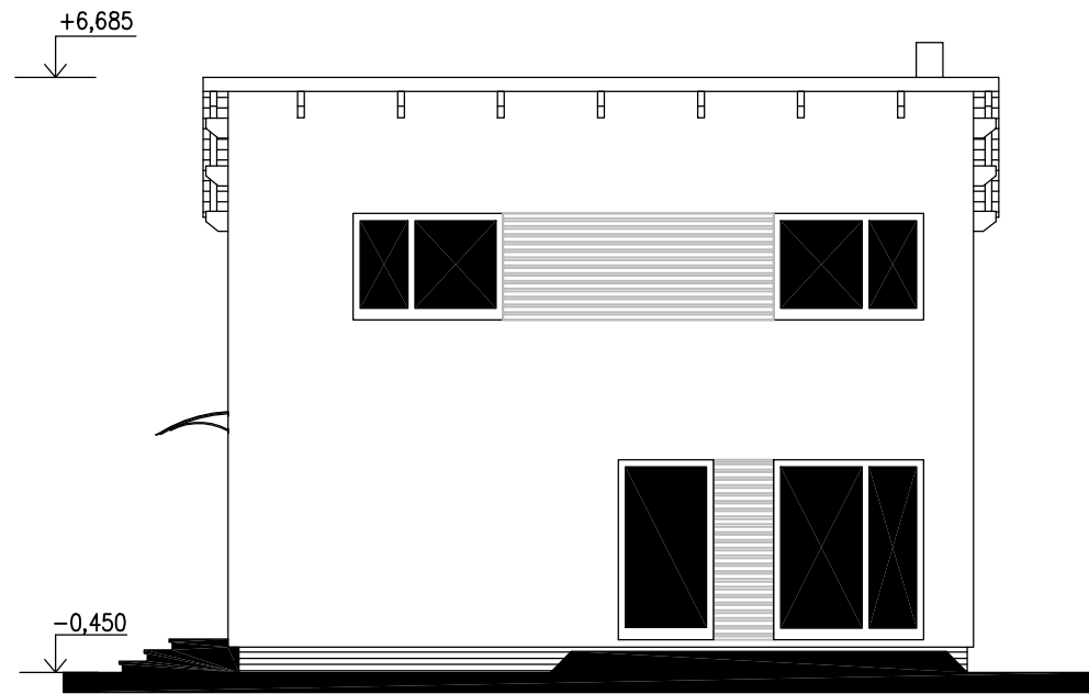
POHLED ZAHRADNÍ
